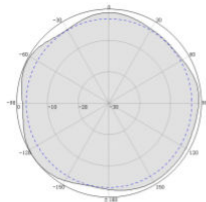
H-Pattern
