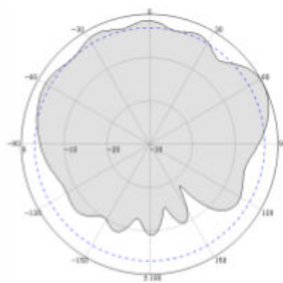
V-Pattern
